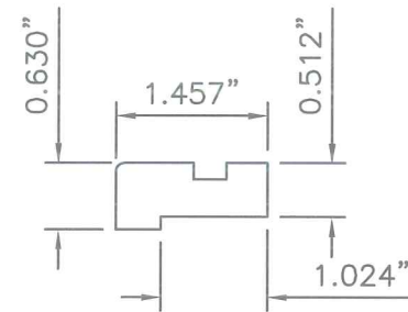
⑦ FILLET (MEETING STILE)
